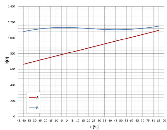
Charakterystyka zależności rezystancji od temperatury (A - CR 1-55, B - CR 1-55-T)
