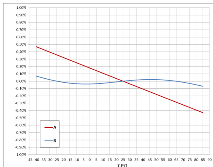
Charakterystyka zależności błęd pomiarowego od temperatury dla R_o=47k\Omega (A - CR 1-55, B - CR 1-55-T)
