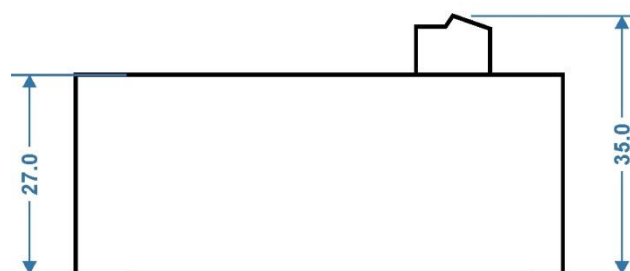
Obudowa CR 1-25, C 1-25-T
