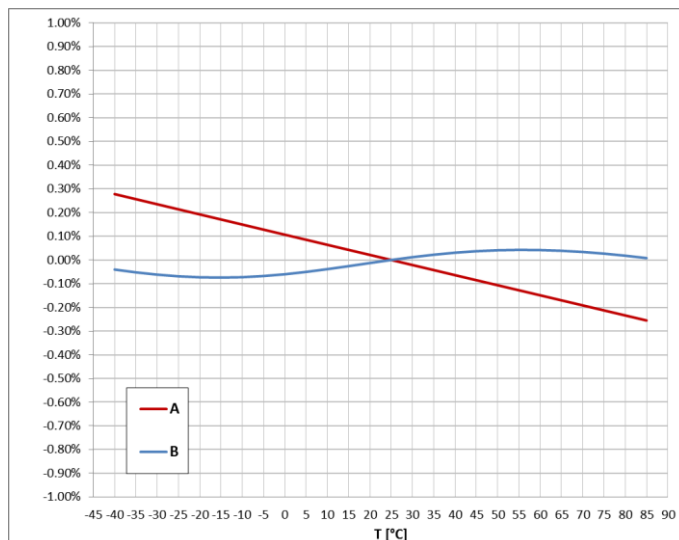
Charakterystyka zależności błędu pomiarowego od temperatury dla R_o=47k\Omega (A - CR 1-25, B - CR 1-25-T)
