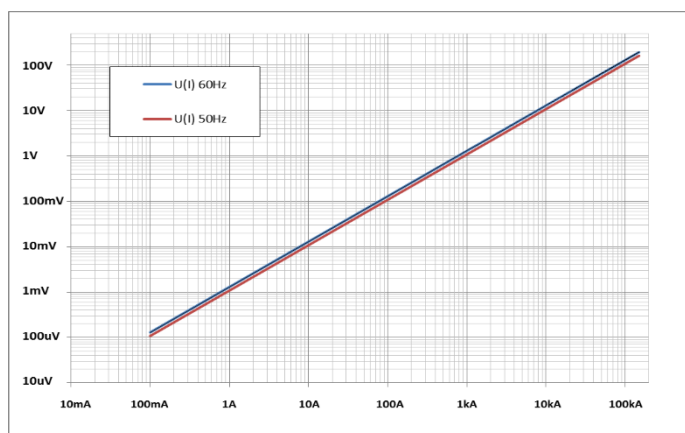
Charakterystyka zależności napięcia wyjściowego U od prądu I
