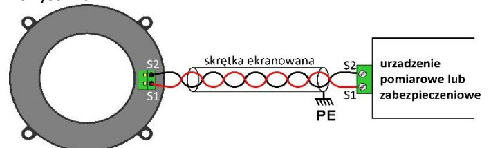
Schemat przyłączeniowy przekładnika CR
