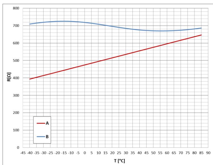
Charakterystyka zależności rezystancji od temperatury (A - CR 1-25, B - CR 1-25-T)
