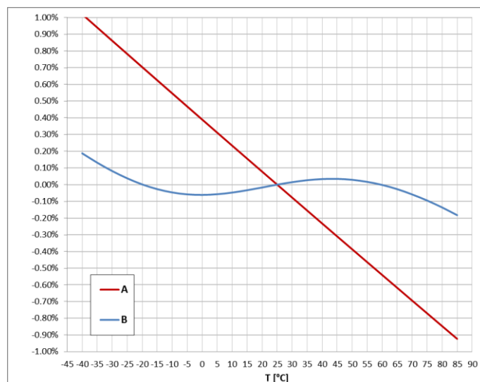
Charakterystyka zależności błędu pomiarowego od temperatury dla R_0=47k\Omega (A - CRR 3-50, B - CRR 3-50-T)
