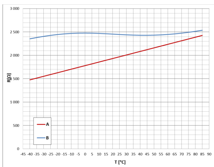
Charakterystyka zależności rezystancji od temperatury (A - CRR 3-50, B - CRR 3-50-T)
