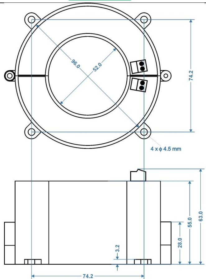
Obudowa CRR 3-50, CRR 3-50-T
