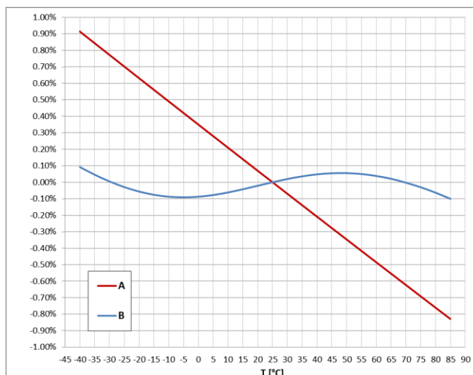
Charakterystyka zależności błędu pomiarowego od temperatury dla R_o=47k\Omega (A - CR 2-55, B - CR 2-55-T)
