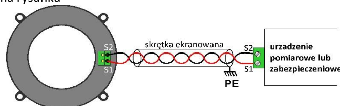
Schemat przyłączeniowy przekładnika CR
