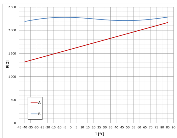
Charakterystyka zależności rezystancji od temperatury (A - CR 2-55, B - CR 2-55-T)
