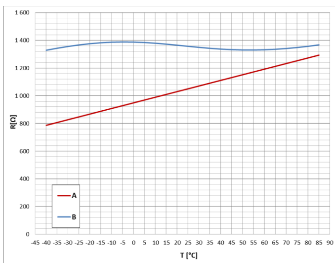
Charakterystyka zależności rezystancji od temperatury (A - CR 2-25, B - CR 2-25-T)
