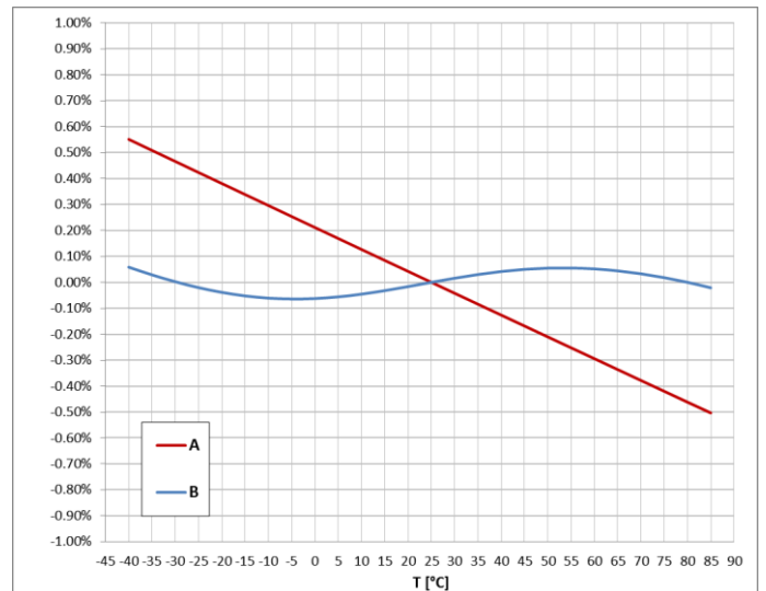
Charakterystyka zależności błędu pomiarowego od temperatury dla R_o=47k\Omega (A - CR 2-25, B - CR 2-25-T)
