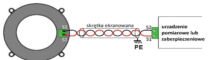
Schemat przyłączeniowy przekładnika CR
