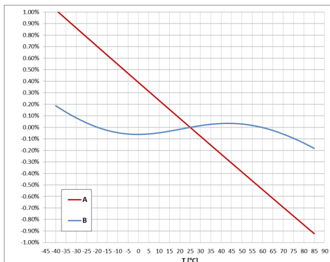
Charakterystyka zależności błędu pomiarowego od temperatury dla R_o=47k\Omega (A - CR 3-50, B - CR 3-50-T)
