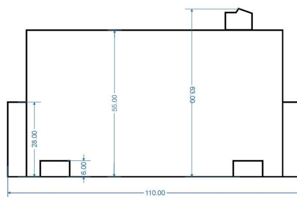
Obudowa CR 3-50, C 3-50-T
