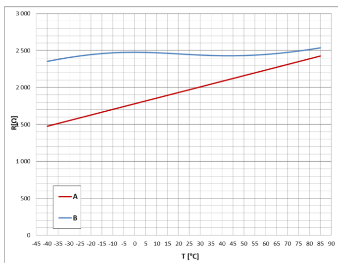
Charakterystyka zależności rezystancji od temperatury (A - CR 3-50, B - CR 3-50-T)
