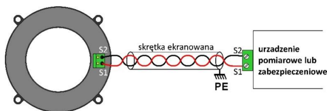
Schemat przyłączeniowy przekładnika CR
