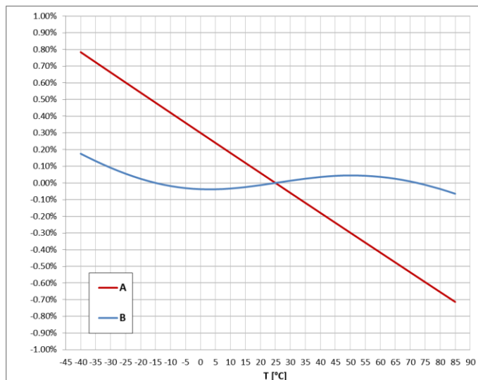
Charakterystyka zależności błęd pomiarowego od temperatury dla R_o=100k\Omega (A - CR 5-50, B - CR 5-50-T)
