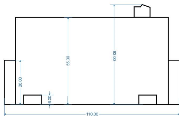
Obudowa CR 5-50, C 5-50-T
