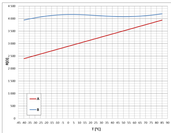
Charakterystyka zależności rezystancji od temperatury (A - CR 5-50, B - CR 5-50-T)
