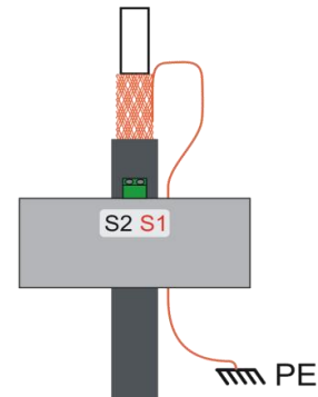
Sposób instalacji przekładnika na kablu prądowym z ekranem
