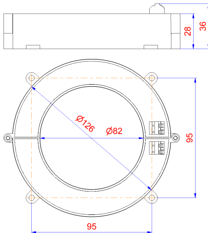
Obudowa CRR 1-80, CRR 1-80-T
