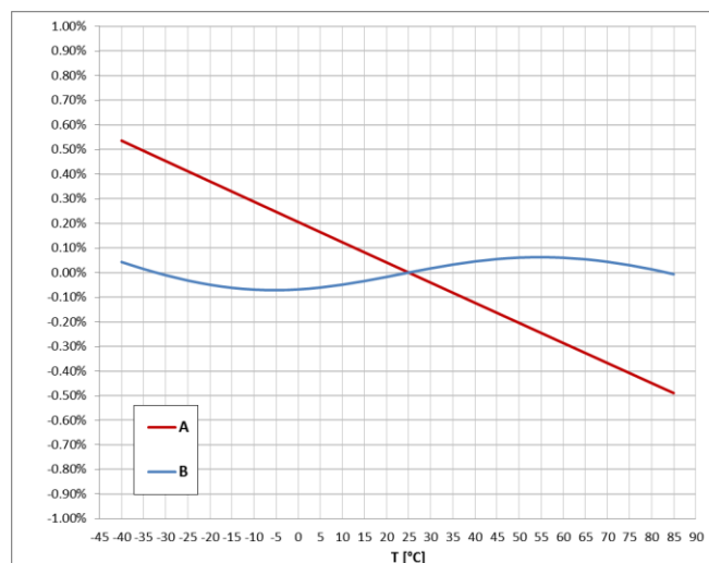
Charakterystyka zależności błęd pomiarowego od temperatury dla R_o=47k\Omega (A - CRR 1-80, B - CRR 1-80-T)
