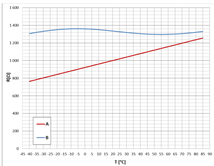
Charakterystyka zależności rezystancji od temperatury (A - CRR 1-80, B - CRR 1-80-T)
