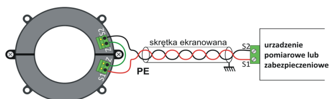
Schemat przyłączeniowy przekładnika CRR
