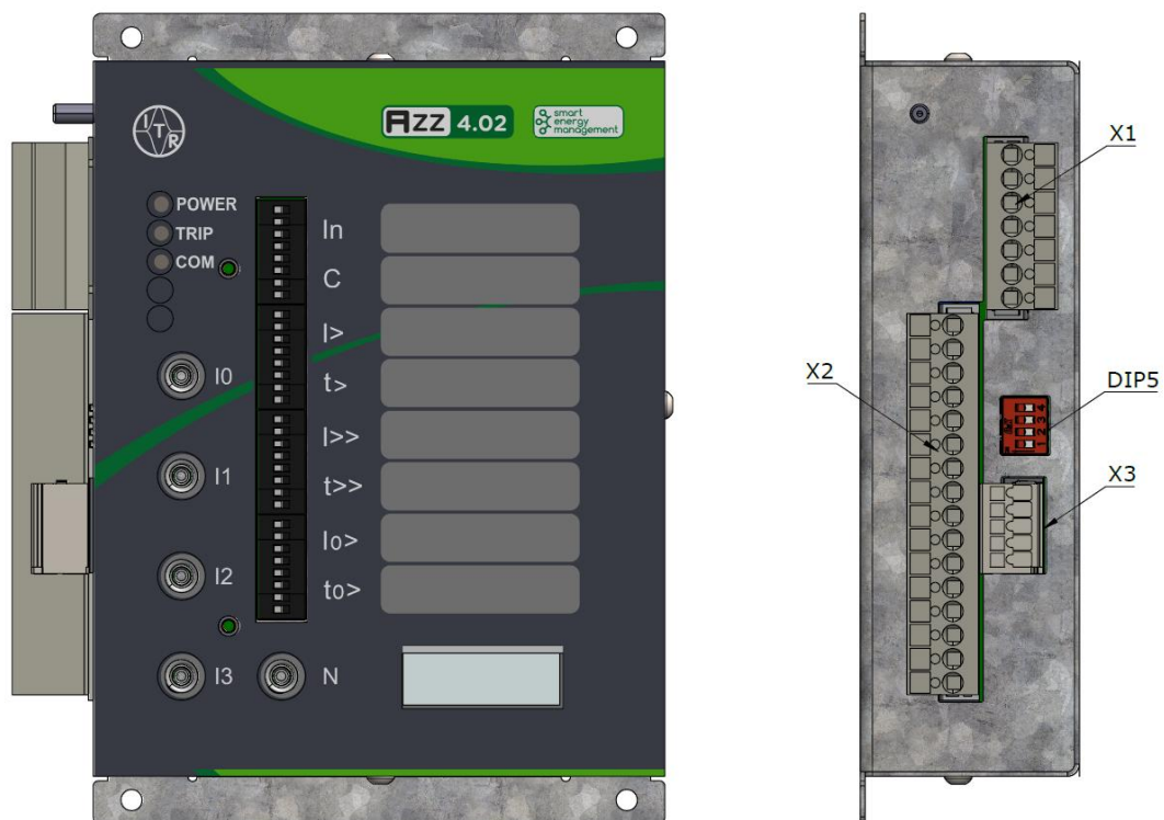
Rys. 9.1. Widok urządzenia od strony złącz
