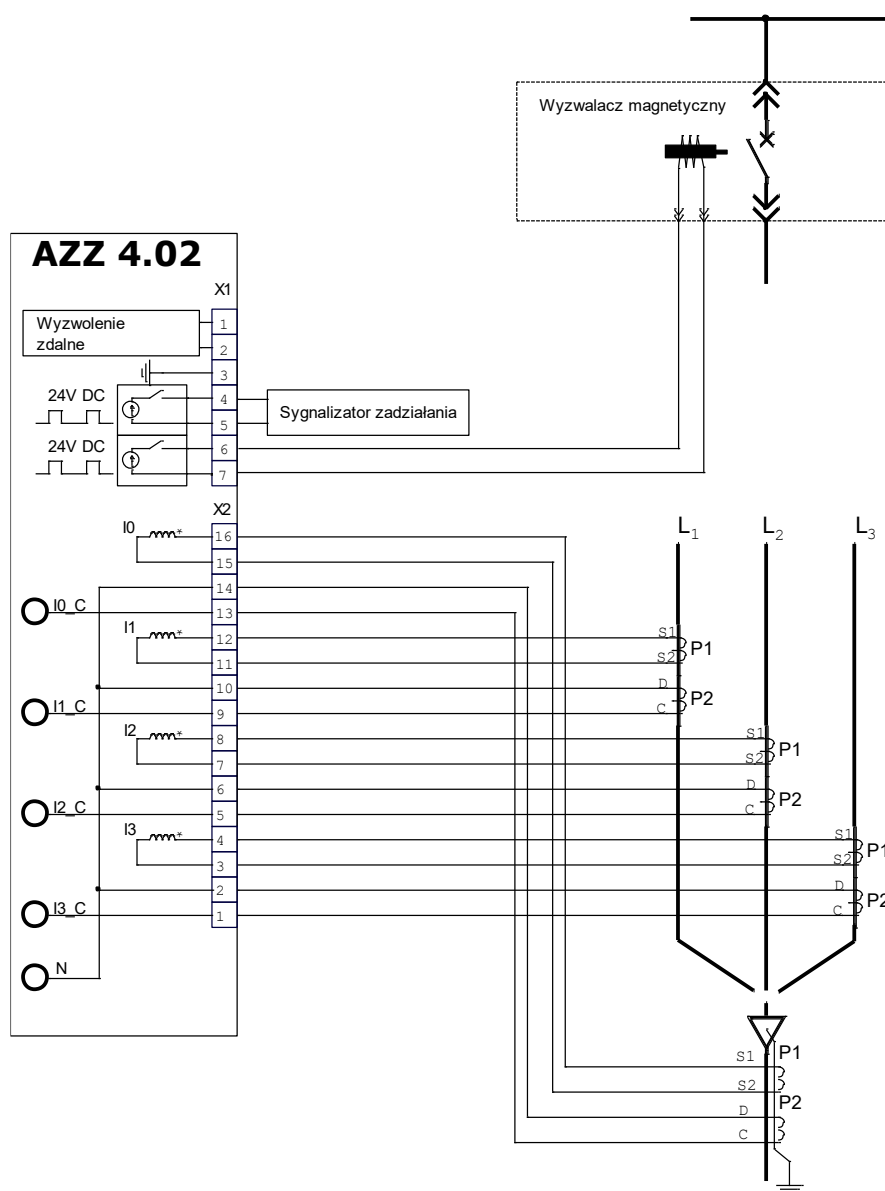
Rys. 8.1. Schemat przyłączeniowy AZZ 4. XX
