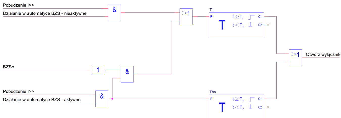
Rysunek 21.3. Algorytm zabezpieczenia szyn w polu łącznika szyn.
