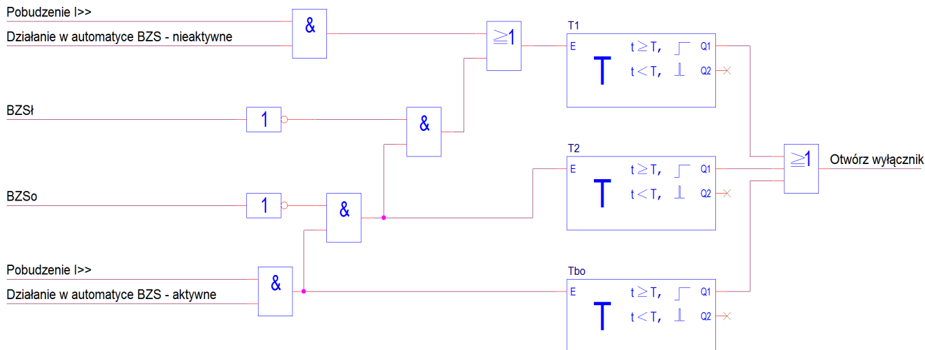
Rysunek 21.2. Algorytm zabezpieczenia szyn w polu zasilającym.
