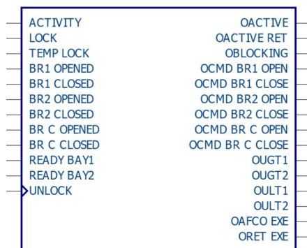
Rysunek 66.1. Blok funkcyjny A_AFCO14_01_01
