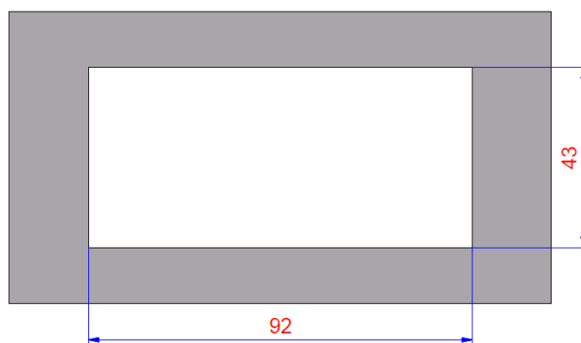
Rys. 8.2. Wymiary otworu montażowego VDIS
