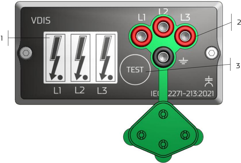
Rys. 2.3.1. Widok płyty czotowej
