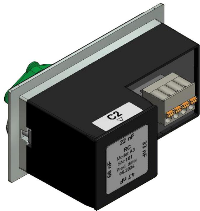
Rys. 9.3. Sposób umieszczenia modułu RC w urządzeniu VDIS
