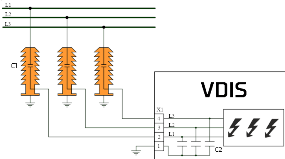
Schemat przyłączeniowy
