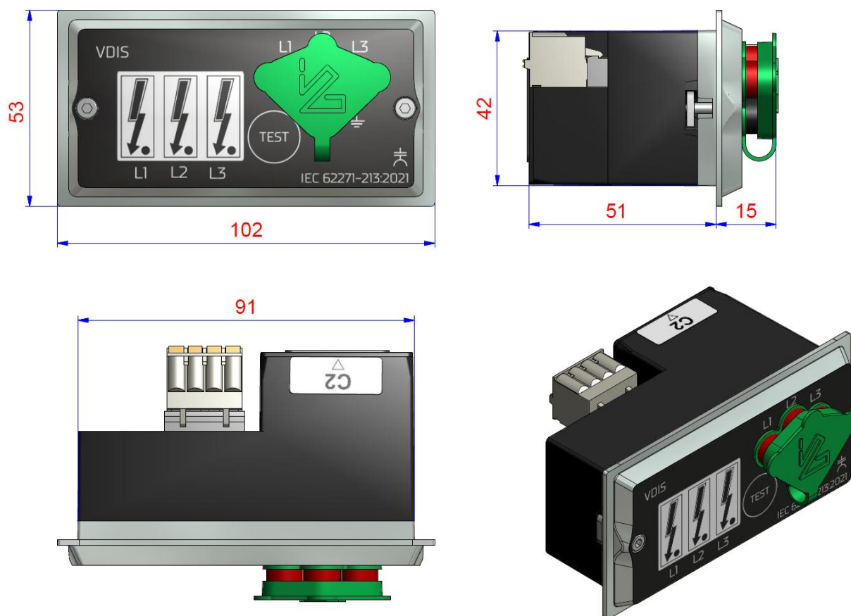
Rys. 8.1. Wymiary urządzenia VDIS
