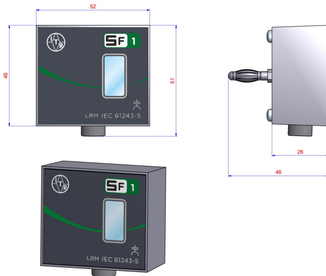
Rys. 8.1. Wymiary obudowy
