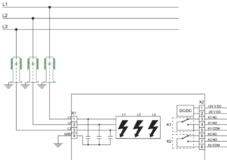
Rys. 7.1. Schemat przyłączeniowy
