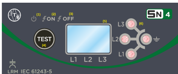
Rys. 2.3.1. Widok płyty czołowej
