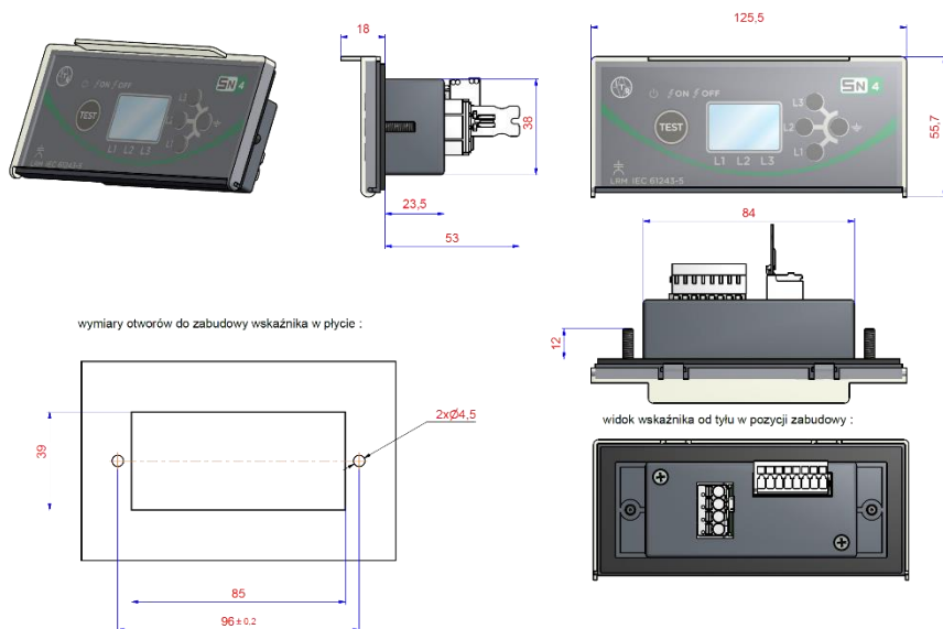
Rys. 8.1. Wymiary obudowy
