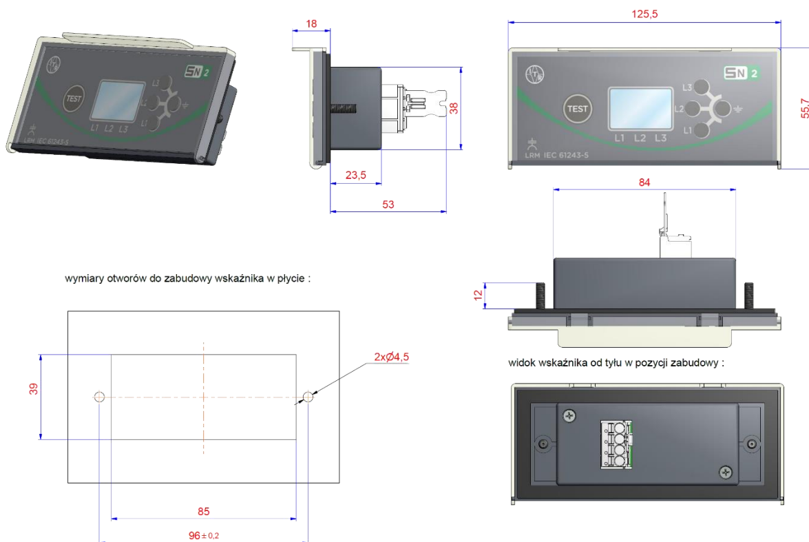
Rys. 8.1. Wymiary obudowy
