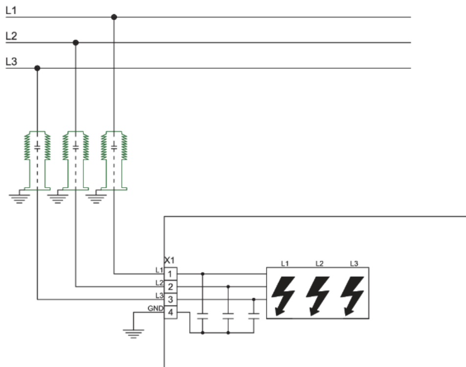
Rys. 7.1. Schemat przyłączeniowy
