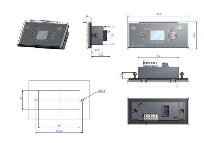
Rys. 8.1. Wymiary obudowy
