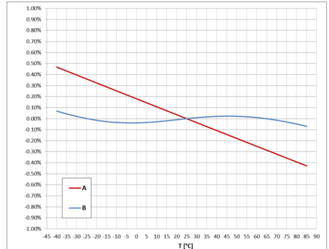
Charakterystyka zależności błędu pomiarowego od temperatury dla R_o=47k\Omega (A - CRR 1-50, B - CRR 1-50-T)
