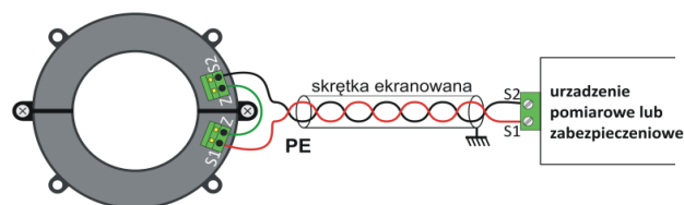
Schemat przyłączeniowy przekładnika CRR
