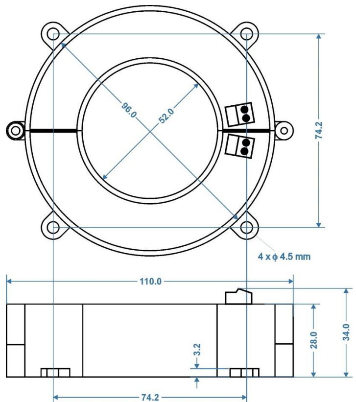
Obudowa CRR 1-50, CRR 1-50-T
