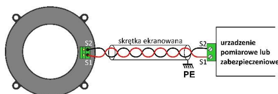
Schemat przyłączeniowy przekładnika CR
