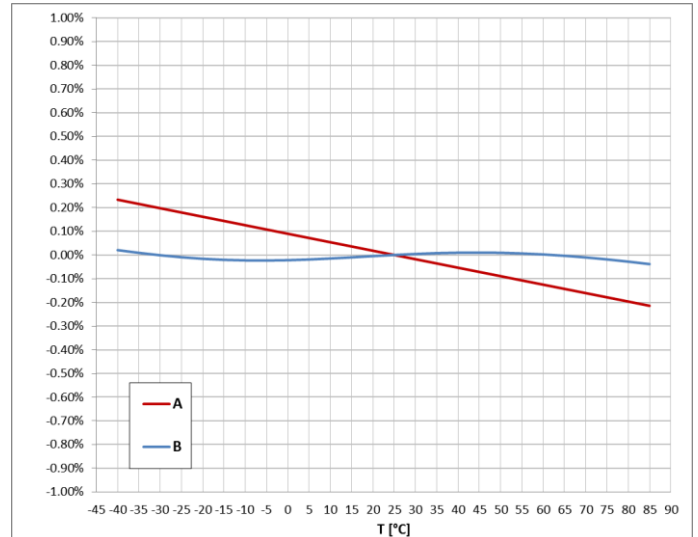
Charakterystyka zależności błęd pomiarowego od temperatury dla R_o=47k\Omega (A - CR 05-55, B - CR 05-55-T)
