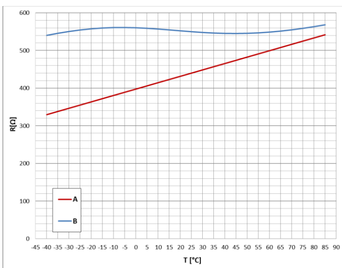
Charakterystyka zależności rezystancji od temperatury (A - CR 05-55, B - CR 05-55-T)
