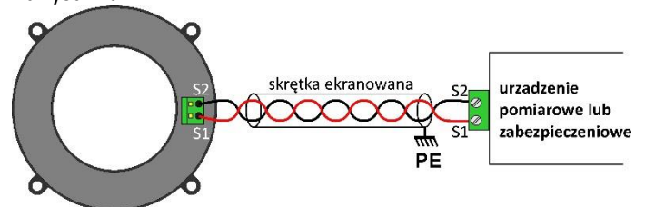
Schemat przyłączeniowy przekładnika CR
