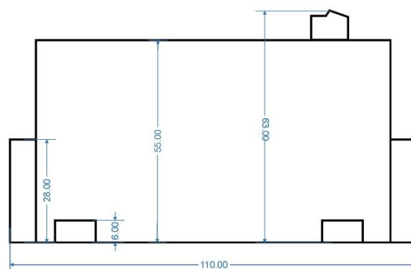
Obudowa CR 6-50, C 6-50-T
