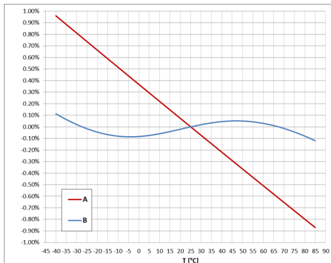
Charakterystyka zależności błędu pomiarowego od temperatury dla R_o=100k\Omega (A - CR 6-50, B - CR 6-50-T)
