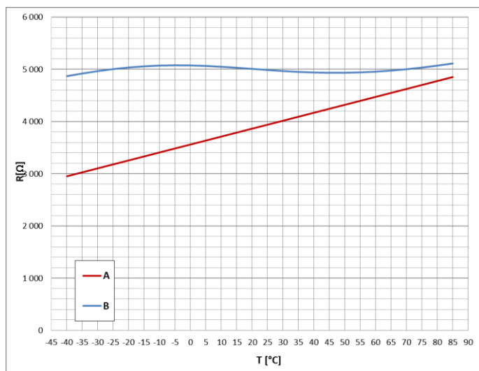
Charakterystyka zależności rezystancji od temperatury (A - CR 6-50, B - CR 6-50-T)
